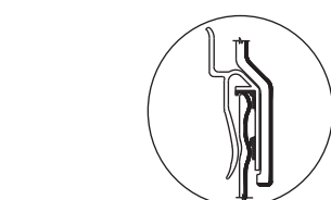
Système « Snap Fit » Can. Patent No. 1240072 Chevauchement sans entretien sur le bain-douche sectionnel.
